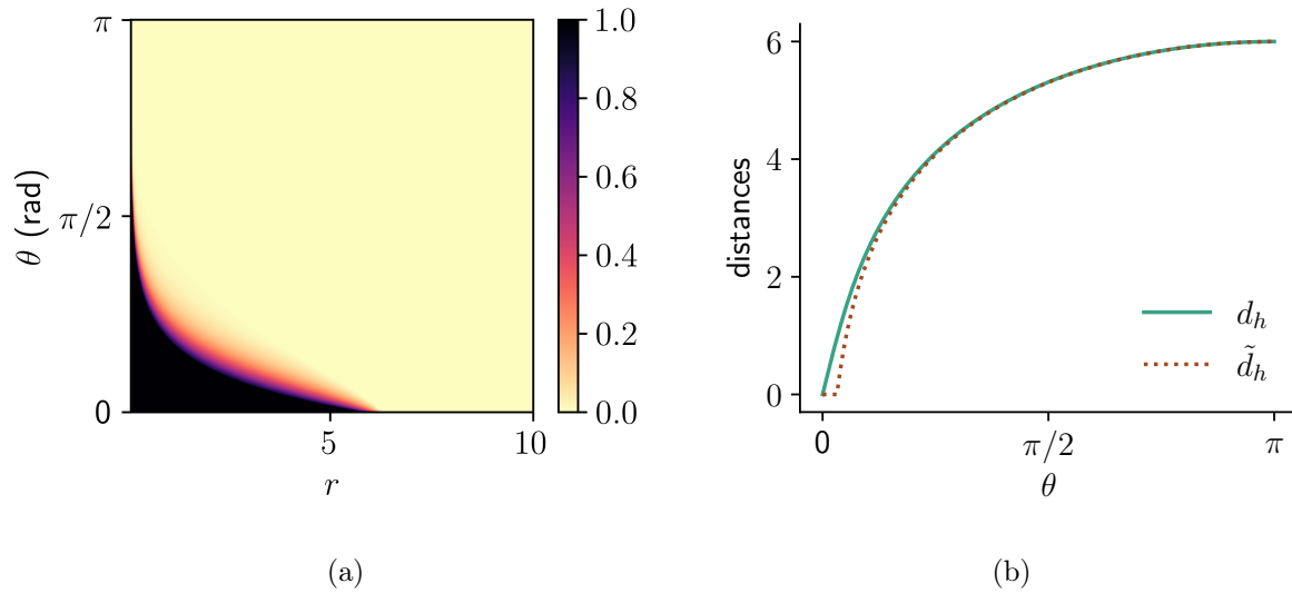
FIGURE 1.8 – Différence entre la distance hyperbolique d_h et son approximation \tilde{d}_h . En (a), l'erreur relative d_h - \tilde{d}_h / d_h est représentée et (b) illustre un exemple de la distance selon la séparation angulaire \theta avec r = r' = 3 .
