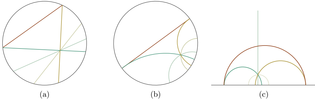
FIGURE 1.5 – Représentations des trois modèles projectifs principaux du plan hyperbolique H^2 . En (a), le disque projectif de Beltrami-Klein, en (b) le disque conforme de Beltrami-Poincaré et en (c) le modèle du demi-plan supérieur de Poincaré. Dans tous les cas, les lignes représentent des géodésiques parallèles.
