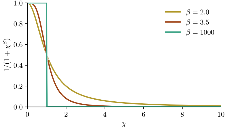
FIGURE 2.3 – Forme générale de la probabilité de connexion selon la valeur du paramètre \beta .
