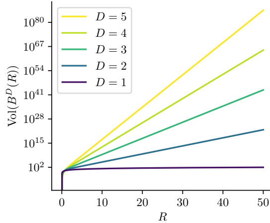
FIGURE 1.7 – Volume D -dimensionnel d'une boule hyperbolique selon la dimension et le rayon R , sur H^D(1) où la courbure est -1 .
